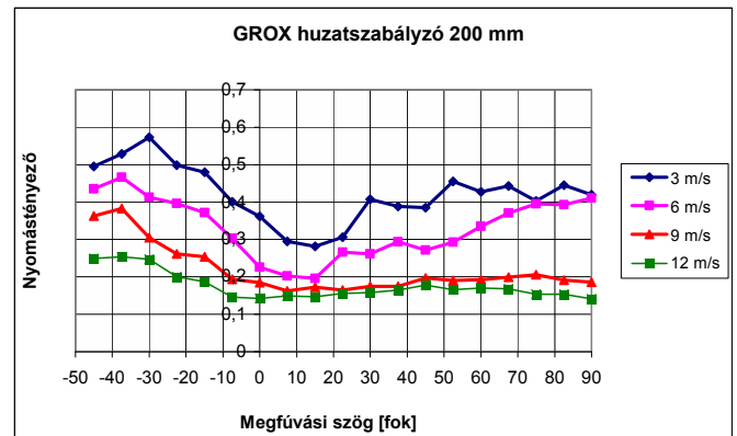
7. ábra A 200 mm-es huzatszabályzó nyomástényezőjének alakulása
